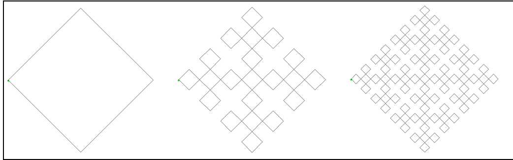
Fig 1 - Kolam con uno, tres y cuatro grados de recursión
